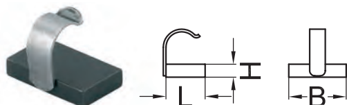
Prism-Longitudinal
